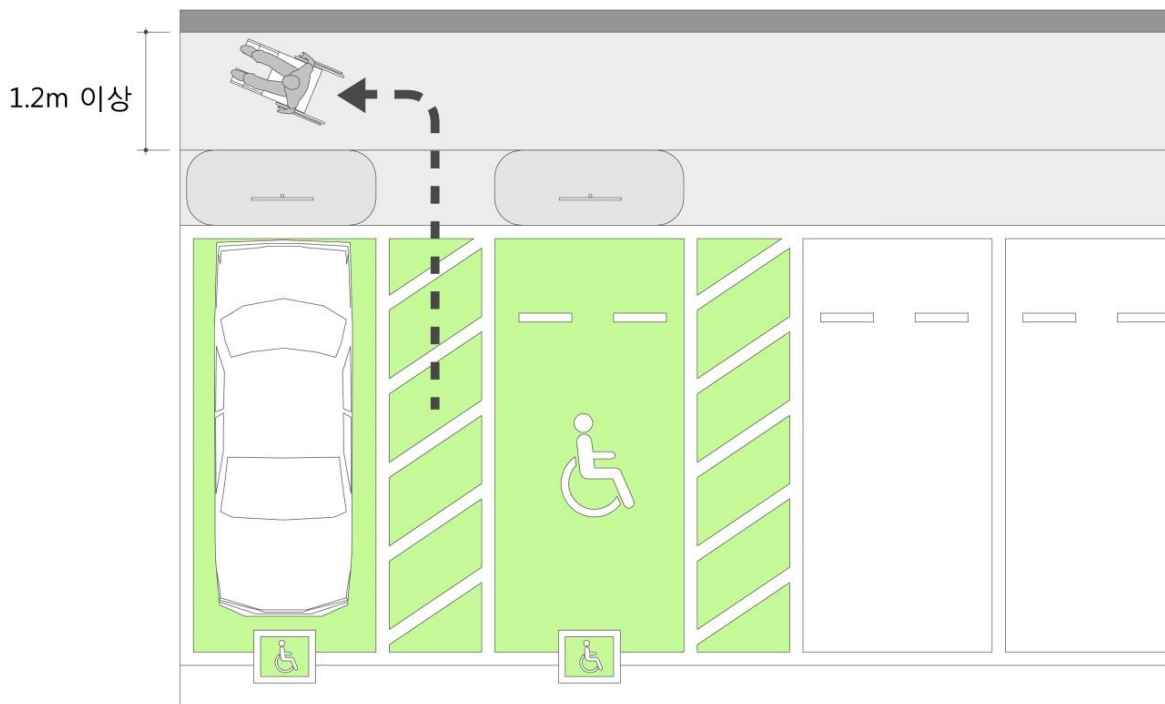
&lt;보행안전통로의 구조&gt;
