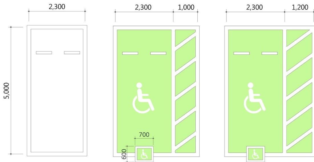
<주차구역의 크기>
