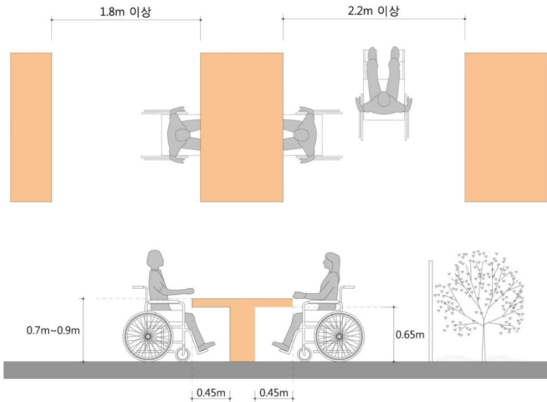
&lt;휴게탁자 구조&gt;
