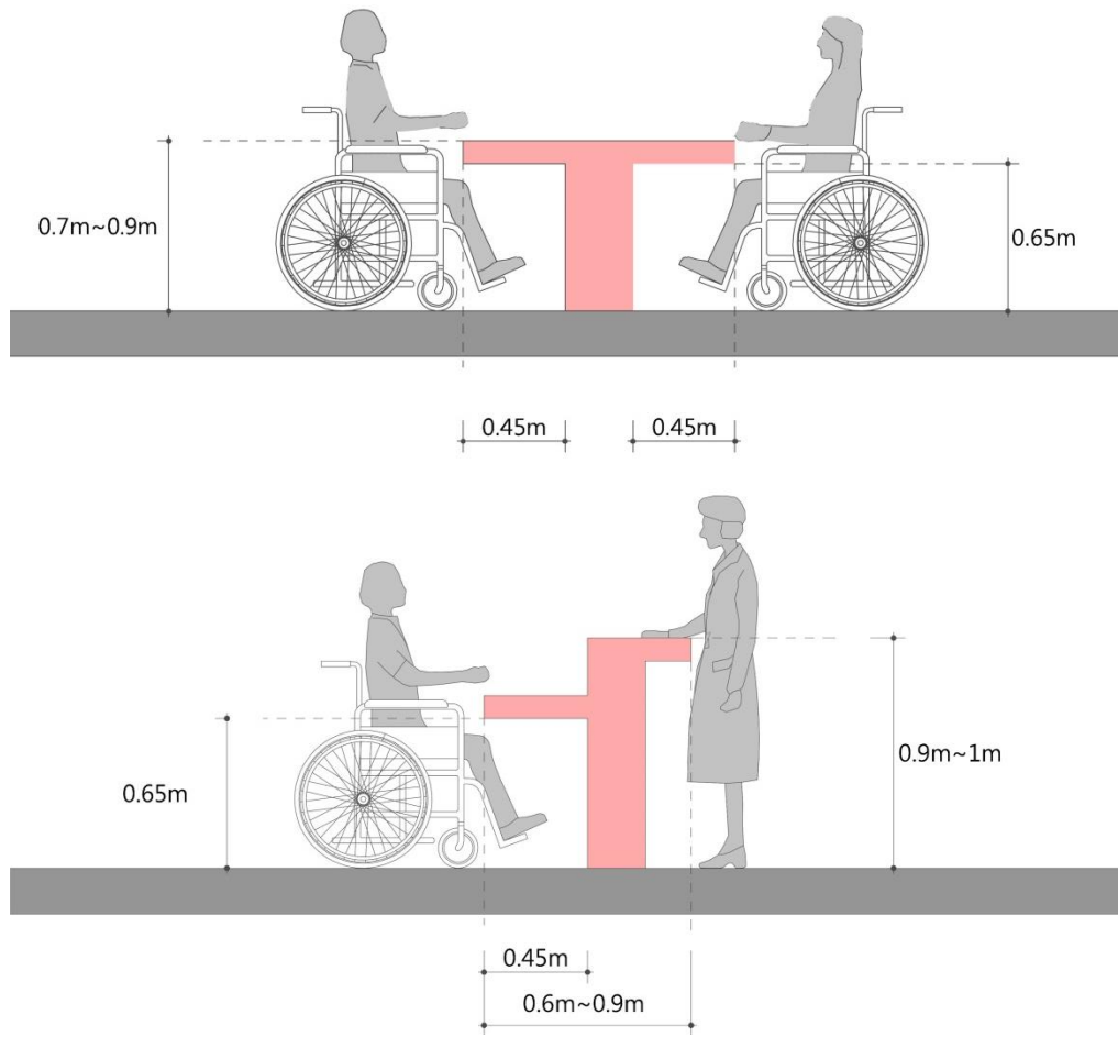
<접수대의 구조>
