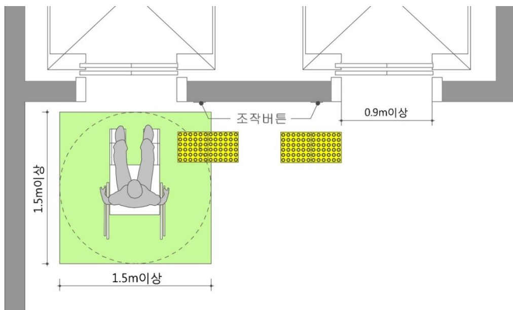
&lt;승강기 출입문 유효폭&gt;
