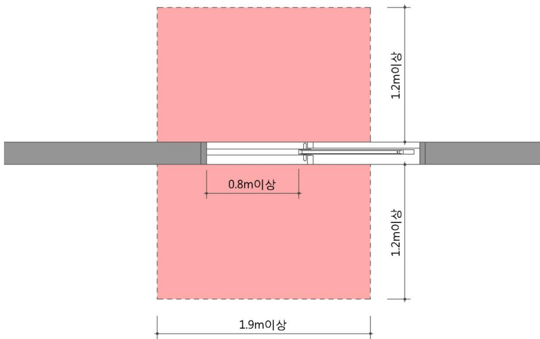
<여닫이문의 활동공간>
