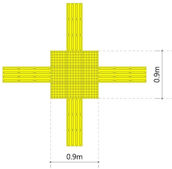
&lt;+자형 교차로&gt;
