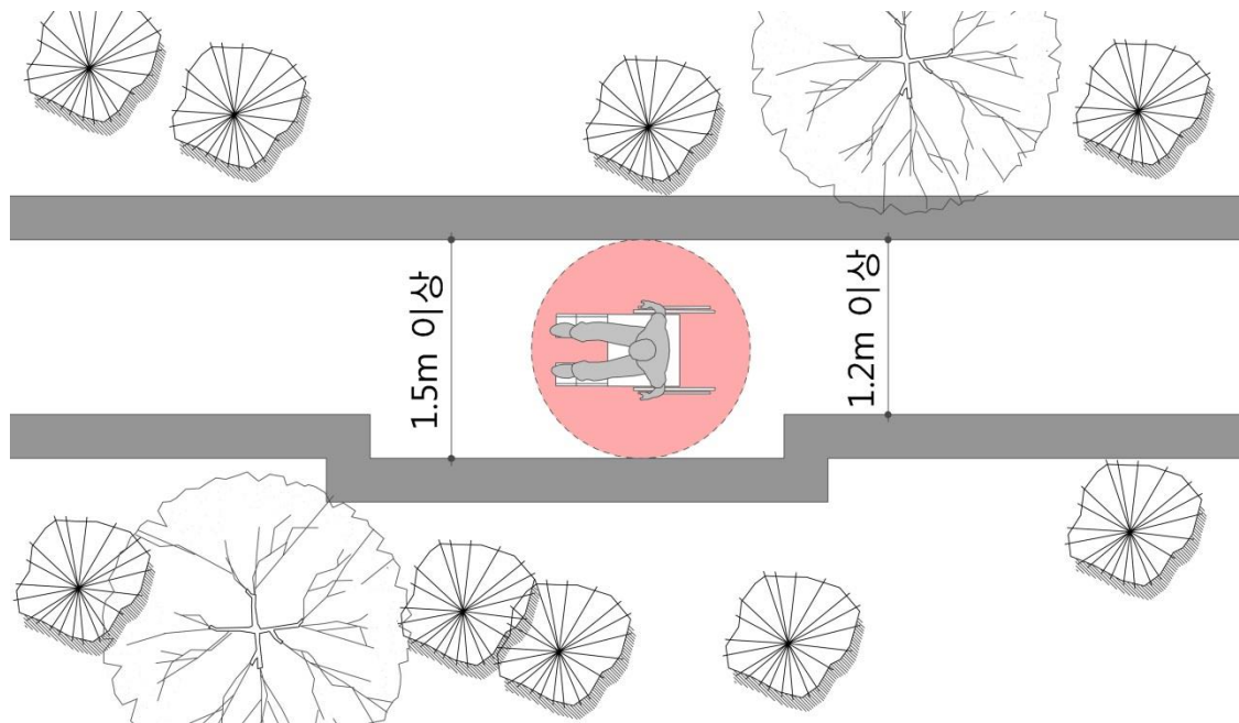
&lt;접근로의 최소 유효폭&gt;
