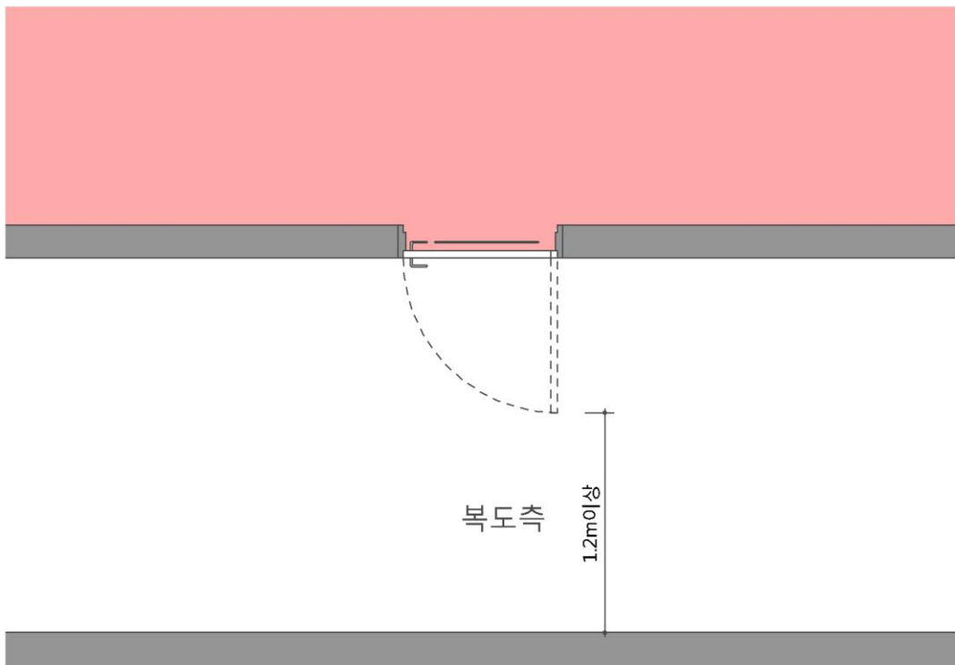
<출입문의 설치방법>
