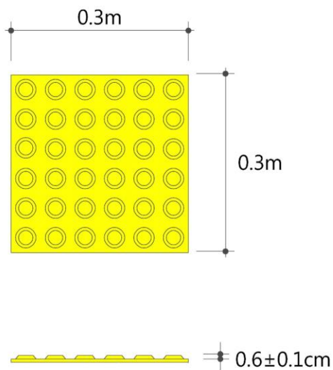
&lt;점형블록&gt;
