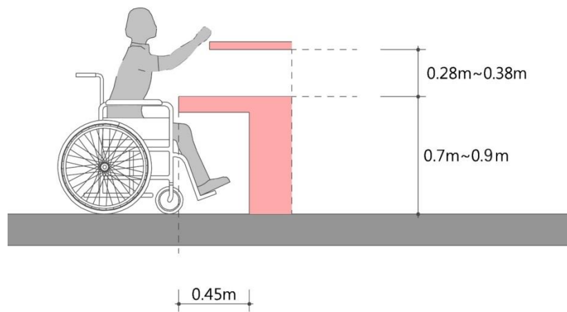
<작업대의 구조>
