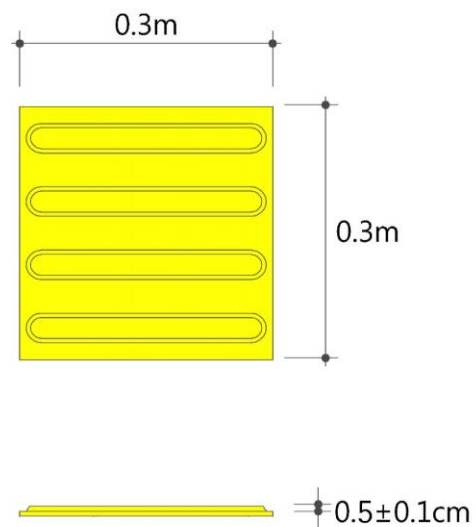
&lt;선형블록&gt;
