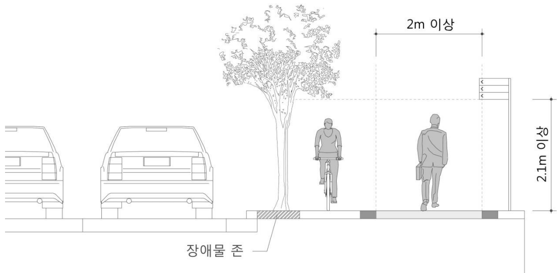
&lt;접근로 유효폭&gt;
