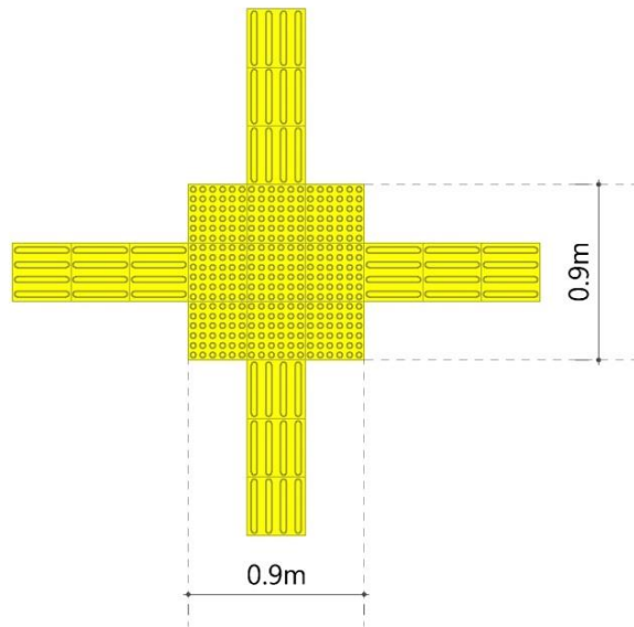
<+자형 교차로>
