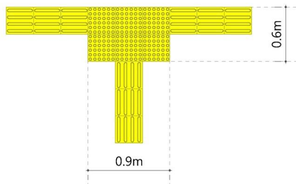
<T자형 교차로>
