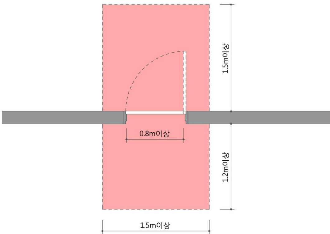
<미닫이문의 활동공간>
