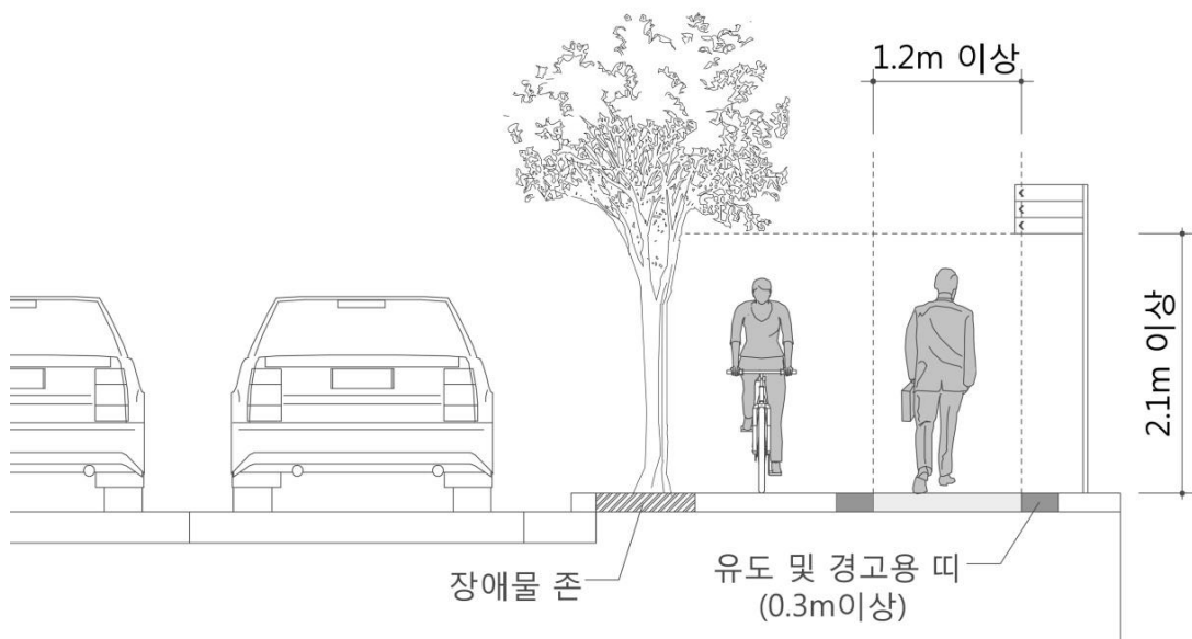
&lt;보행안전통로의 형태&gt;
