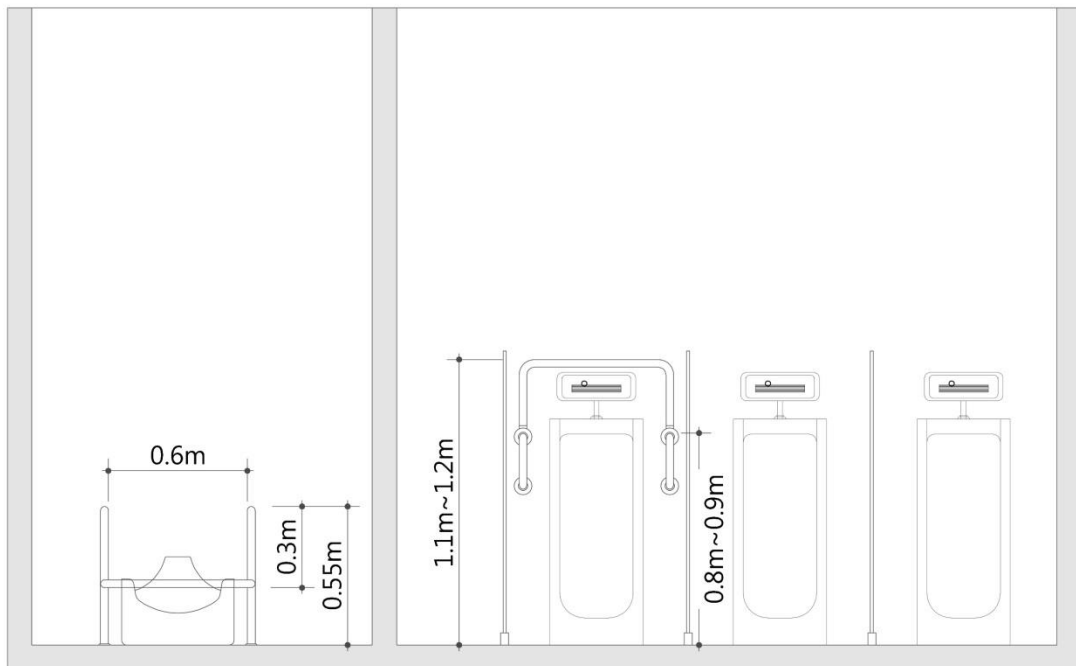
&lt;소변기 소잡이 설치방법&gt;
