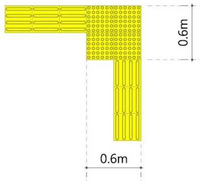
<L자형 교차로>
