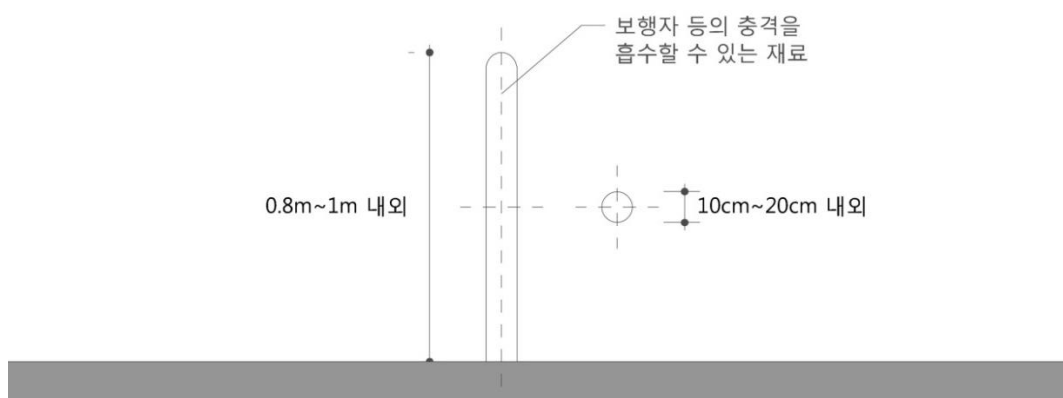
&lt;진출입 통제시설&gt;
