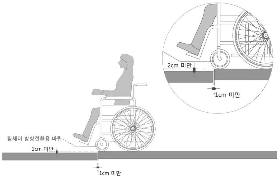
&lt;바닥면 높이차이&gt;
