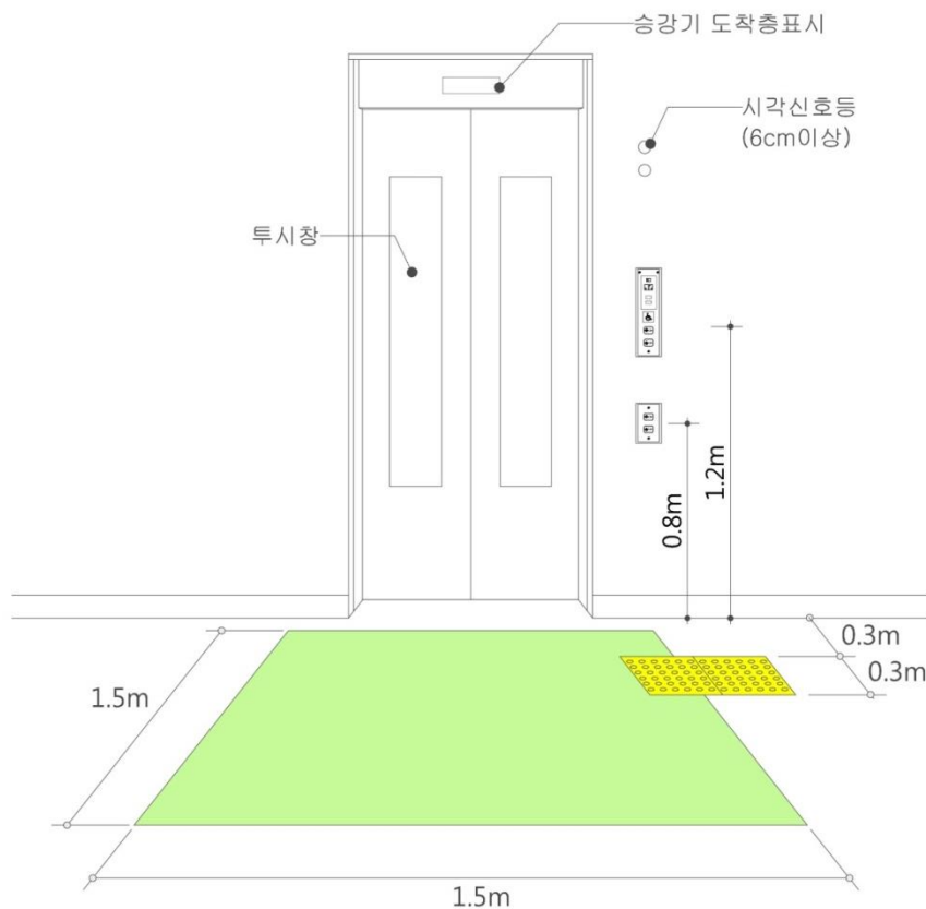
&lt;승강기 전면 활동공간&gt;
