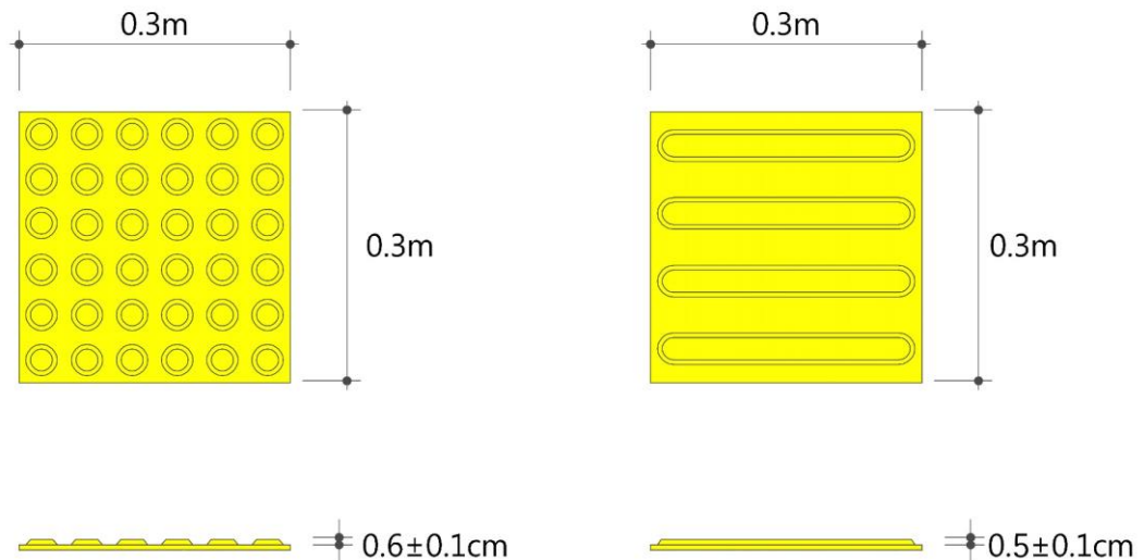
&lt;점자블록의 형태&gt;
