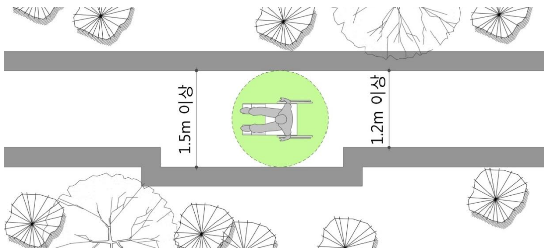
&lt;보행로의 최소 교행공간&gt;
