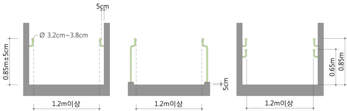
<경사로 유효폭 및 손잡이>
