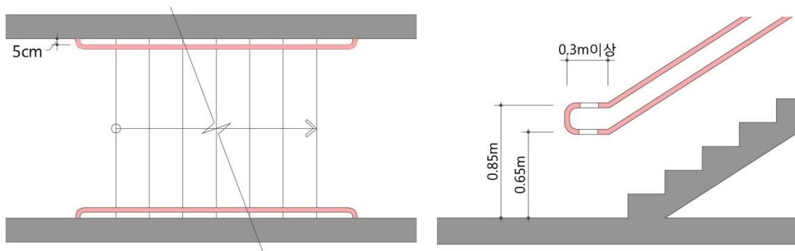
&lt;손잡이 설치방법&gt;
