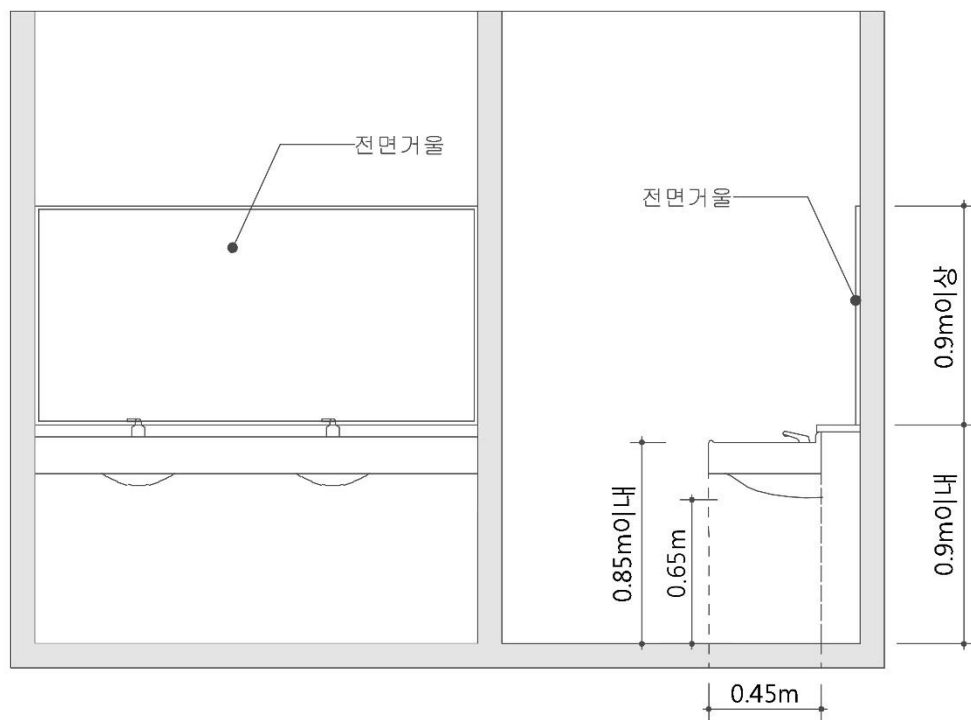
<전면거울 설치>
