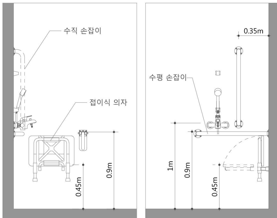
&lt;장애인 등의 이용이 가능한 샤워실&gt;
