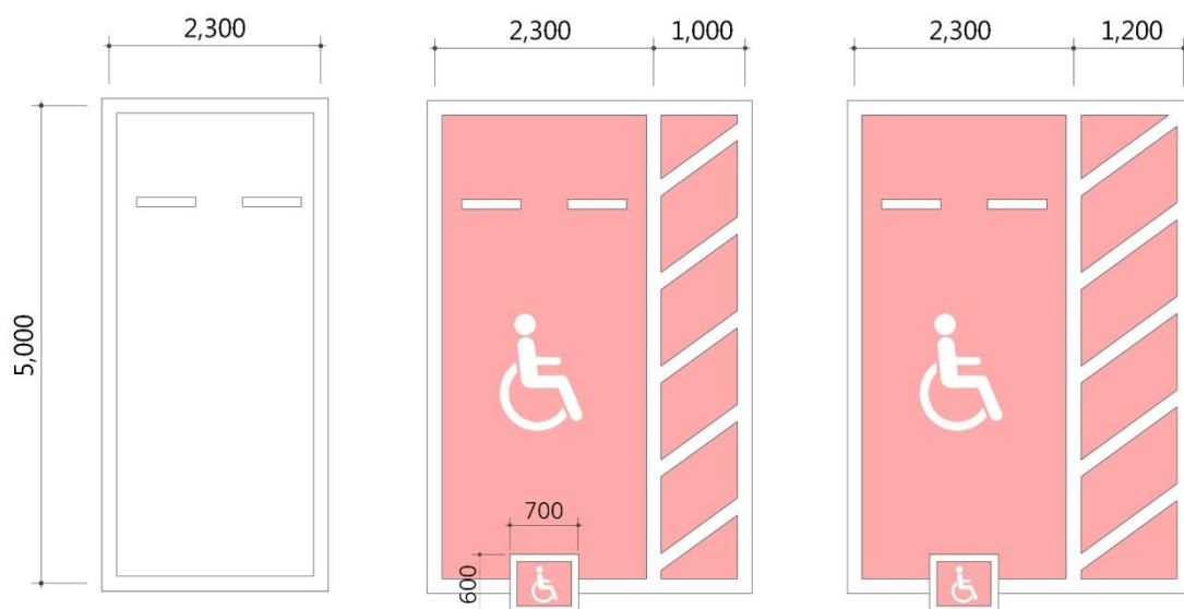
<주차구역의 크기>
