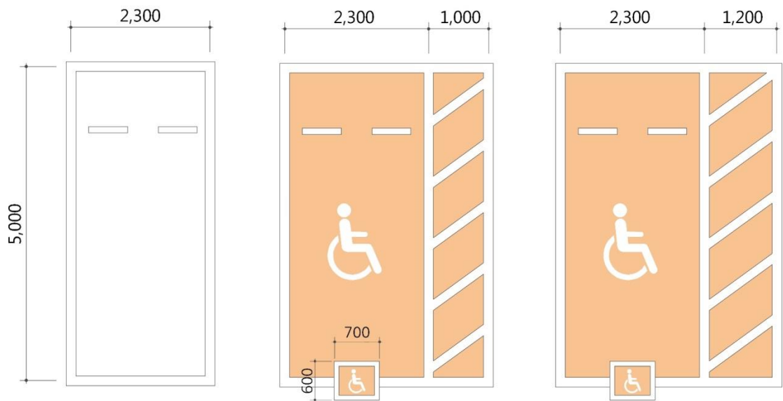
<일반 주차>
