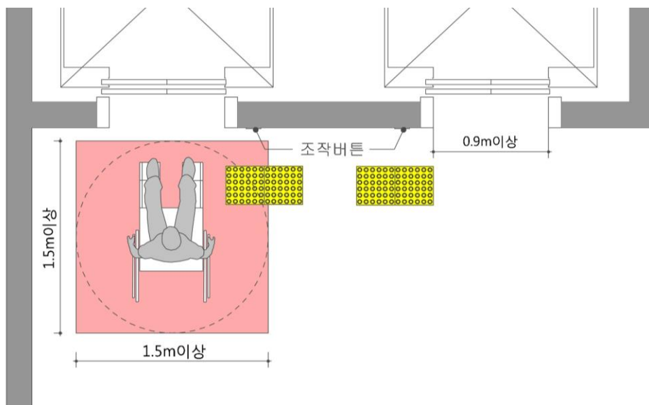
&lt;승강기 출입문 유효폭&gt;
